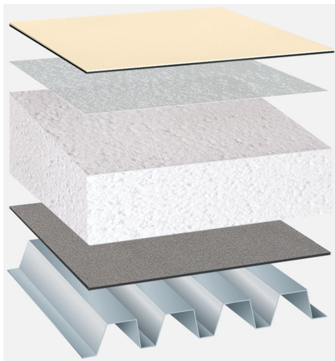
Systemowy układ warstw: TP_EPS-G_T_01
