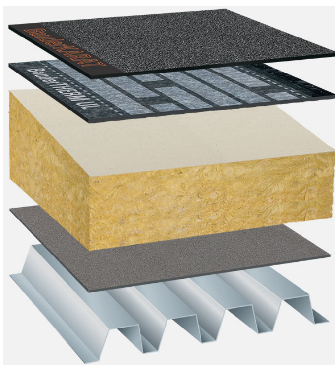
Systemowy układ warstw: TP_MIFA-G_K_01
