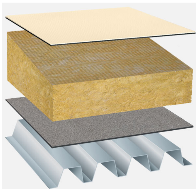
Systemowy układ warstw: TP_MIFA-G_T_01
