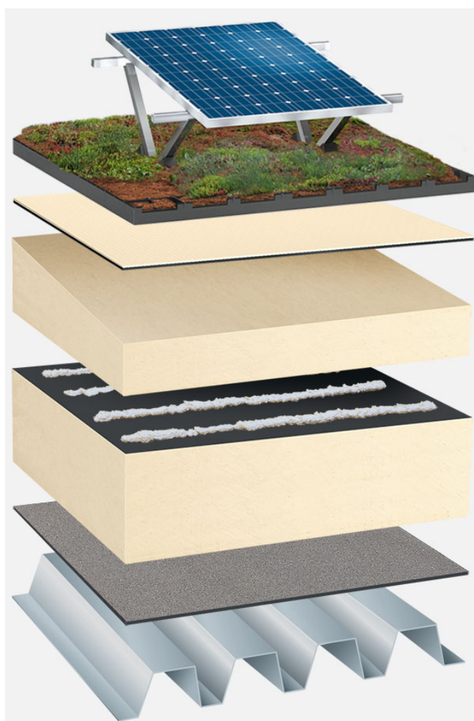
Systemowy układ warstw: TP_PIR-FA_PIR-TG_T_01_PVGD
