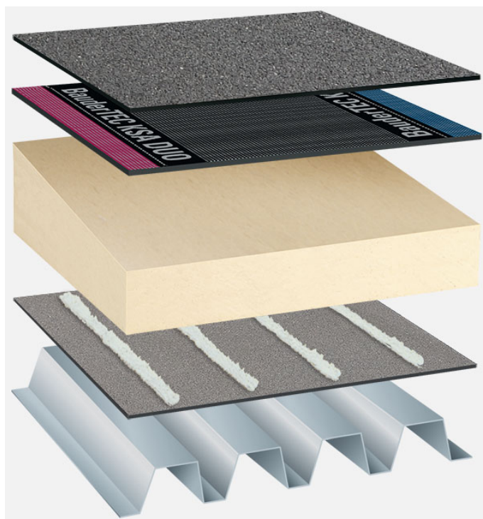
Systemowy układ warstw: TP_PIR-TG_B_01
