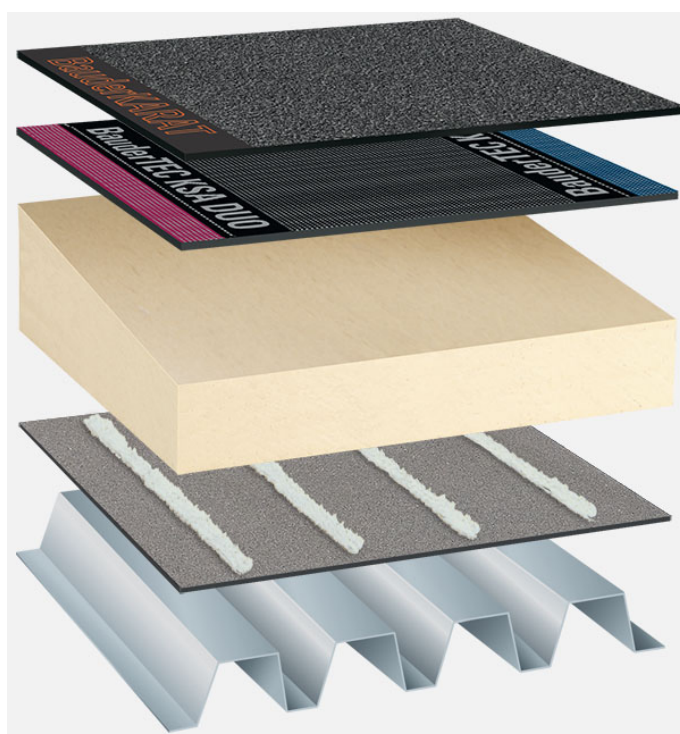
Systemowy układ warstw: TP_PIR-TG_K_01
