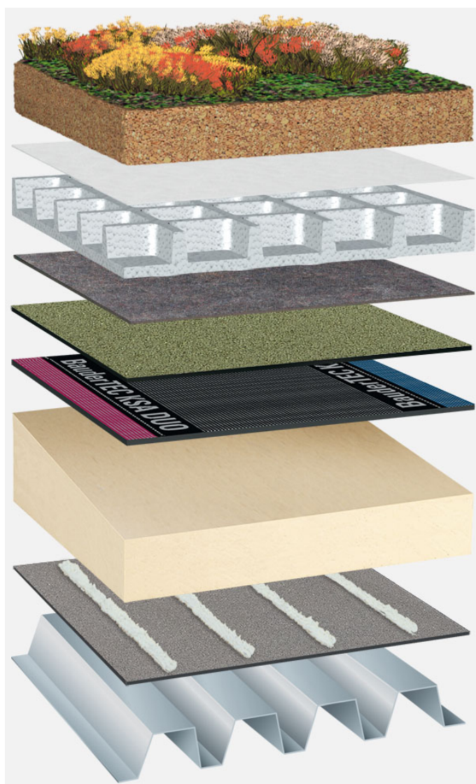
Systemowy układ warstw: TP_PIR-TG_P_01_G75
