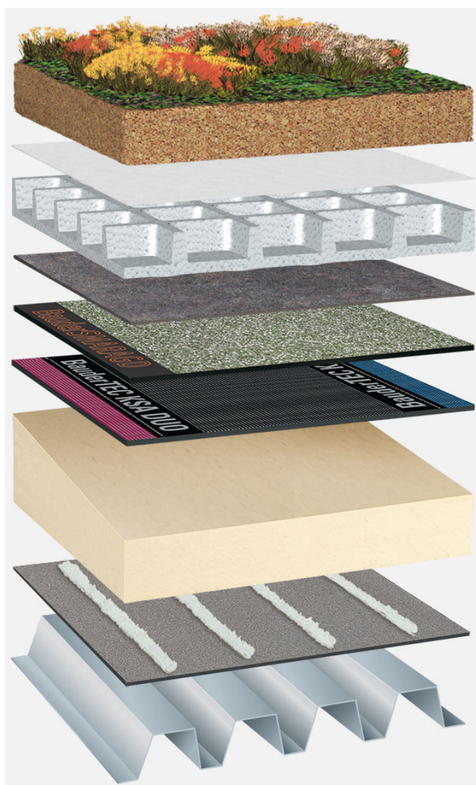
Systemowy układ warstw: TP_PIR-TG_S_01_G75
